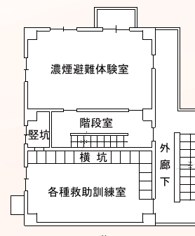
2階平面図
