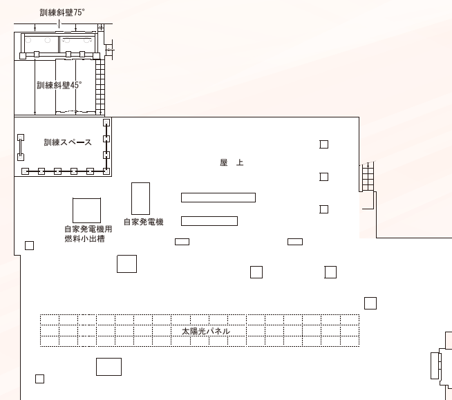
訓練斜壁 45°/75°
